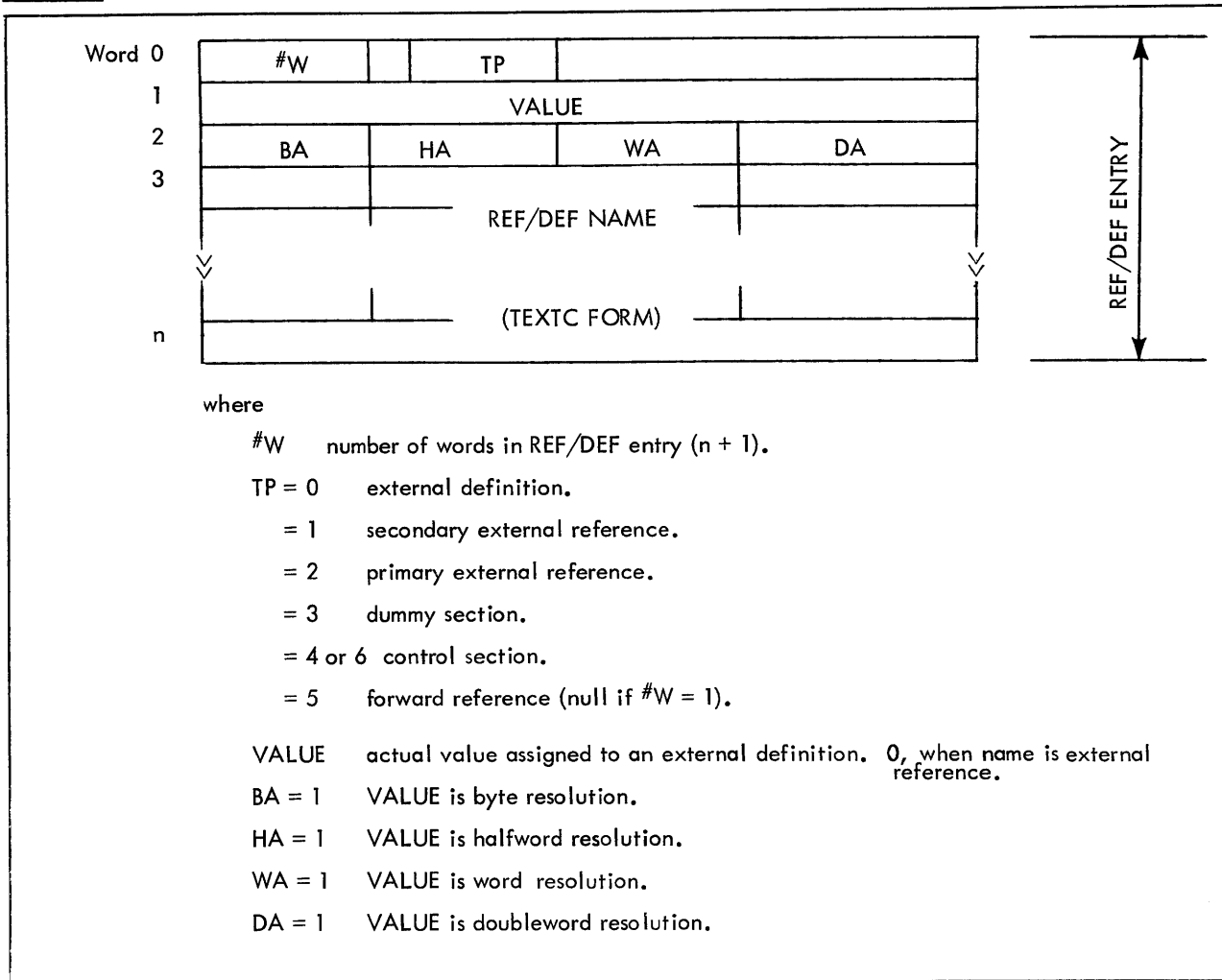
Figure 6-6. RDFSTK Format
